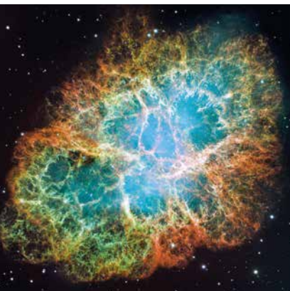
Nébuluse du Crabe.
