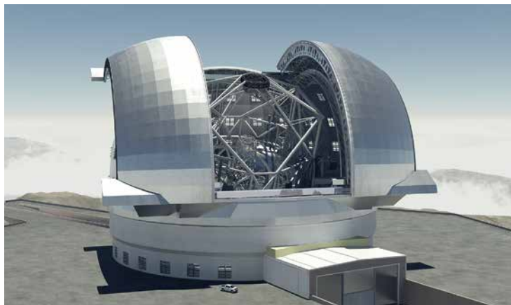
Télescope géant européen, Chili. Vue d'artiste.
